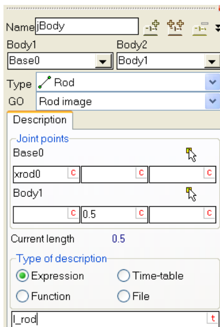
Figure 1.192. Rod joint parameters
