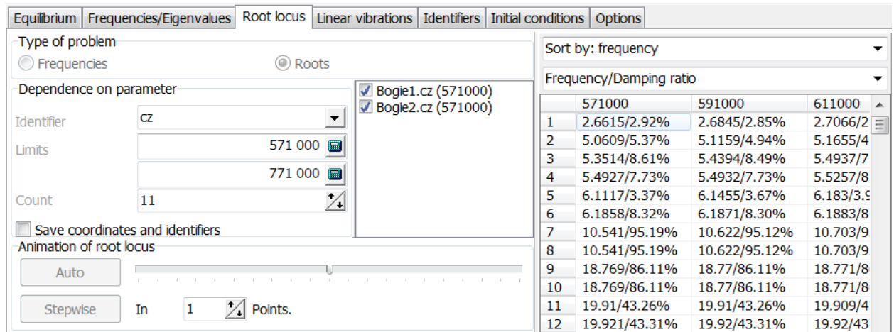
Figure 1.148. EVs vs parameter cz
