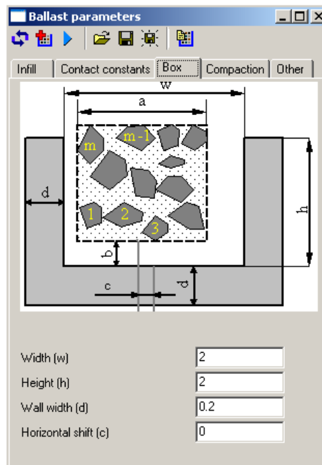
Figure 1.6. Ballast parameters dialog.
