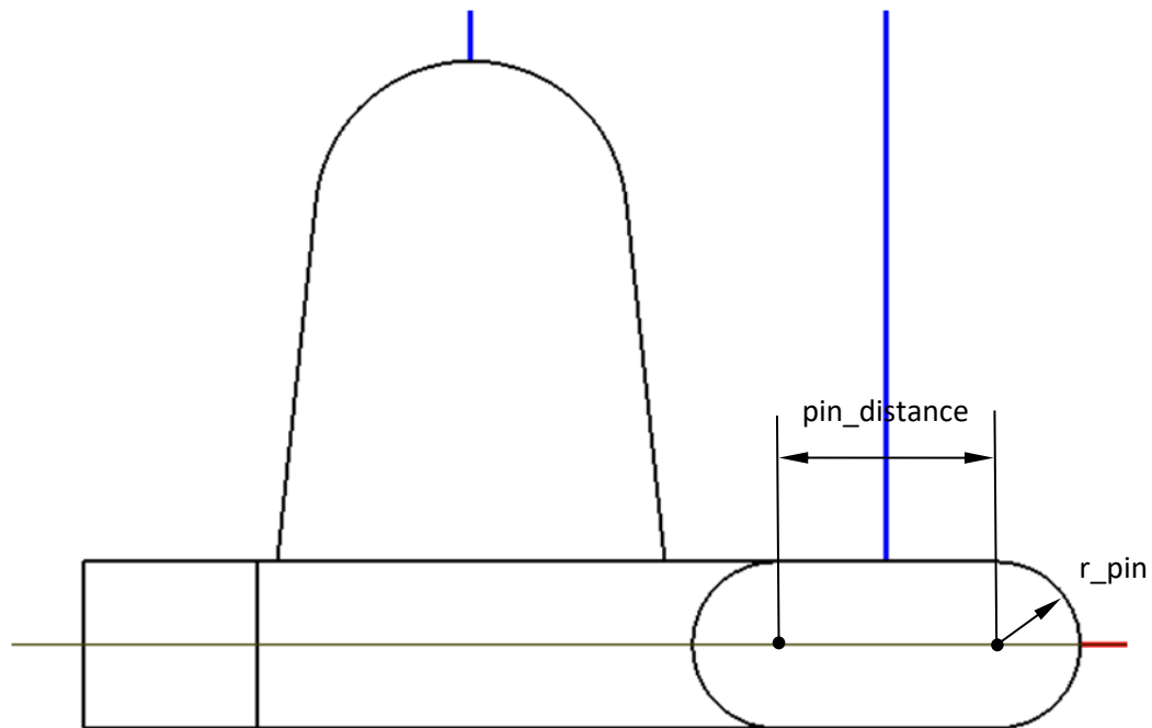
Figure 1.65. Geometrical parameters
