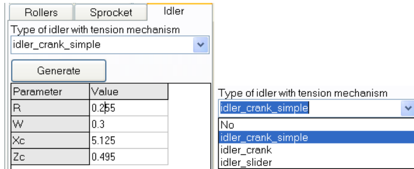
Figure 1.88. Idler parameters
