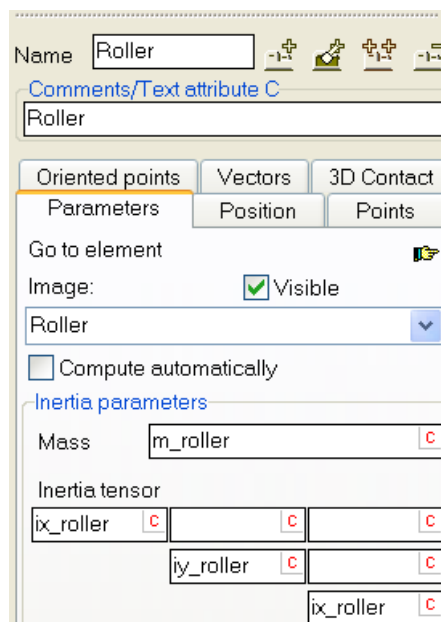
Figure 1.67. Roller body parameters
