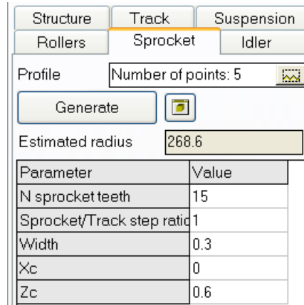
Figure 1.86. Sprocket parameters
