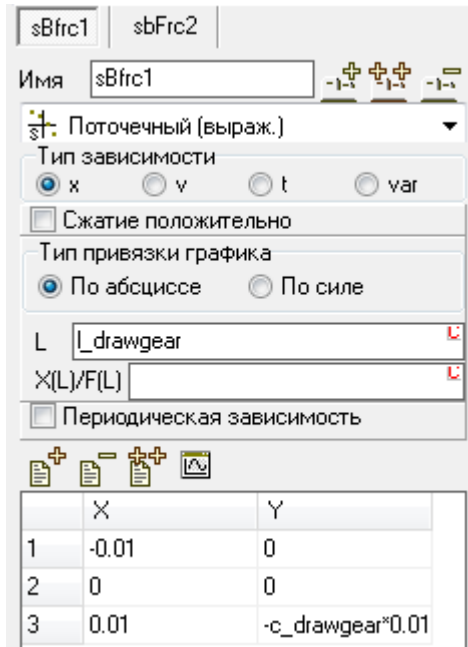
Рис. 1.37. Внешний элемент: продольная тяга, работающая на растяжение. Упругая составляющая
