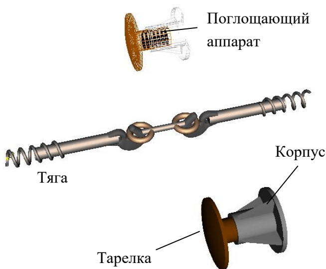
Рис. 1.31. Схема элементов модели буферного сцепного устройства
