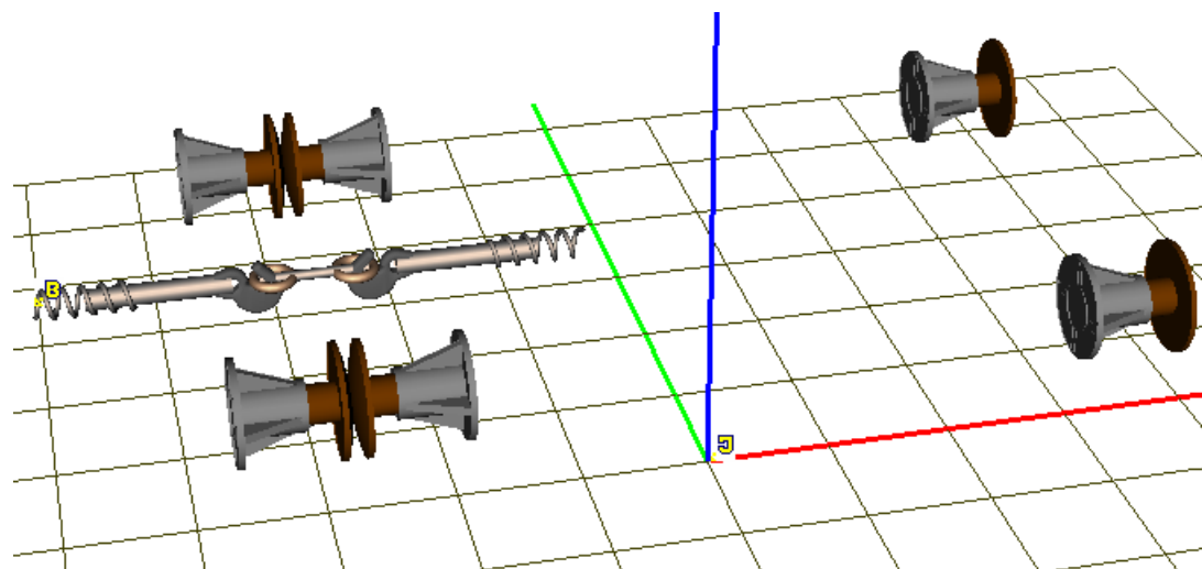
Рис. 1.27. Модель буферного сцепного устройства (объект Buffer_Ext_R )
