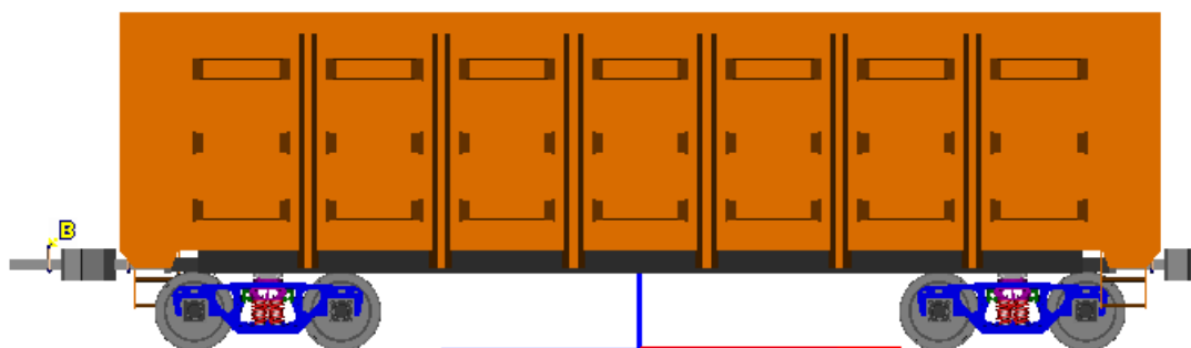
Рис. 1.9. Модель грузового вагона simple_18_100_AC_ExtR , оборудованного автосцепным устройством по модели AC_Standard_EXT_R
