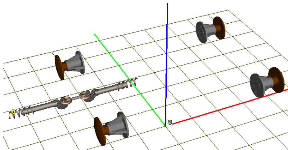
Рис. 1.25. Модель элементов буферного сцепного устройства (объект Buffer )
