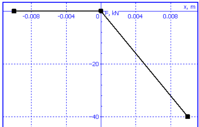
Рис. 1.37. Внешний элемент: продольная тяга, работающая на растяжение. Упругая составляющая
