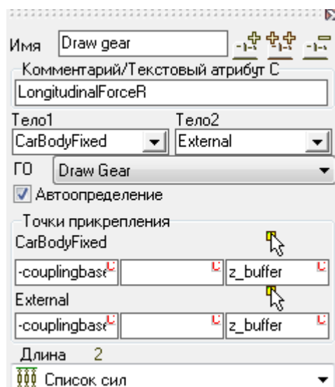
Рис. 1.36. Продольная тяга
