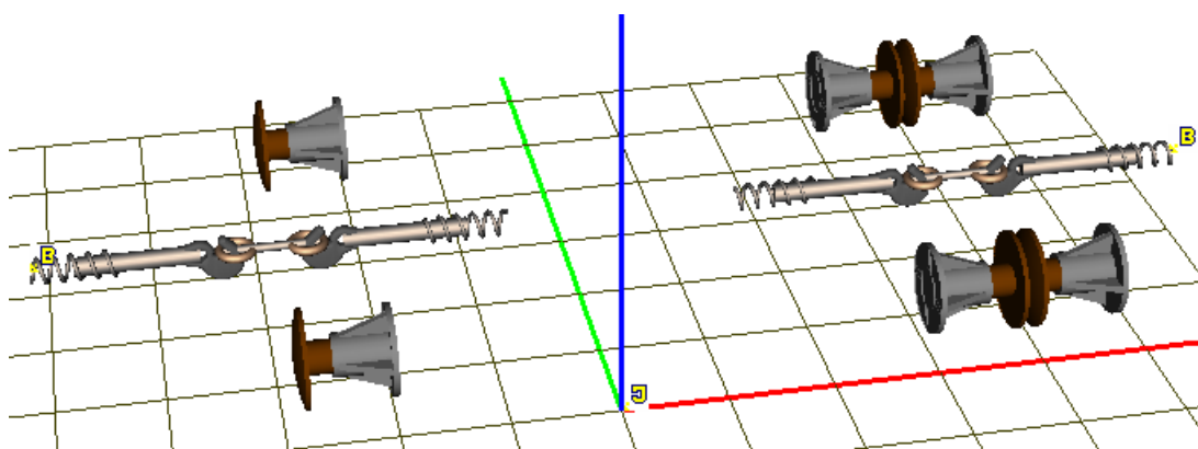
Рис. 1.26. Модель буферного сцепного устройства (объект Buffer_Ext_F )
